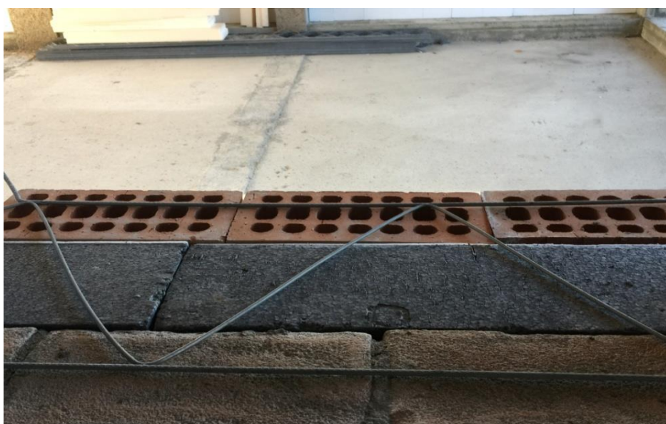
LEGATURA DELLE MURATURE CON RETE con apposita rete murfort
