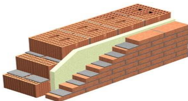
LEGATURA DELLE MURATURE CON RETE con apposita rete murfort
